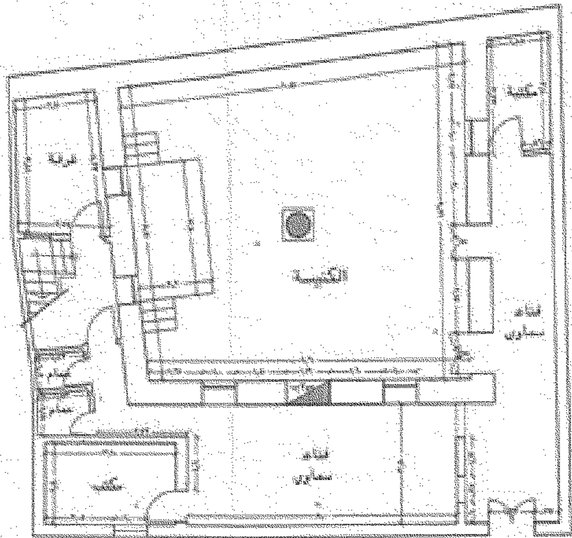
مخطط القسط الأرضي مقياس الرسم ١/٥٠
